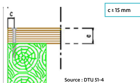
Coupe longitudinale sur lames de platelage jointoient en bout / mur
