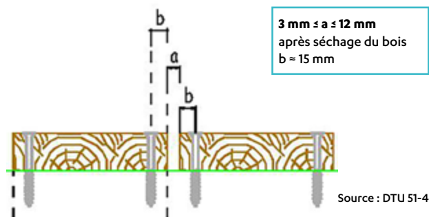
Coupe transversale sur lames de platelage
